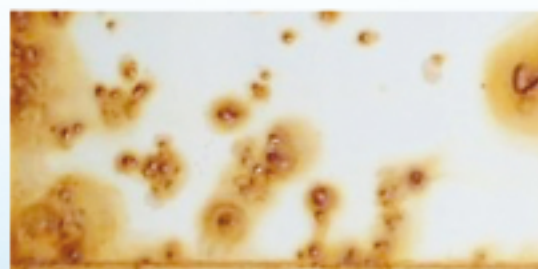
Peinture (2 couches) sur primaire antirouille solvanté (1 couche)
